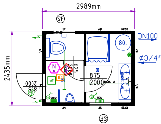
Bungalow sanitaire 10'
