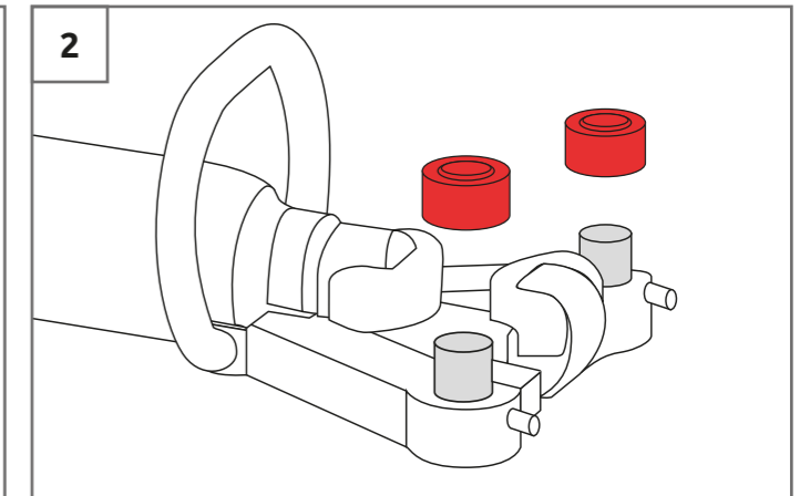
Remove the rollers Togliere le boccole
