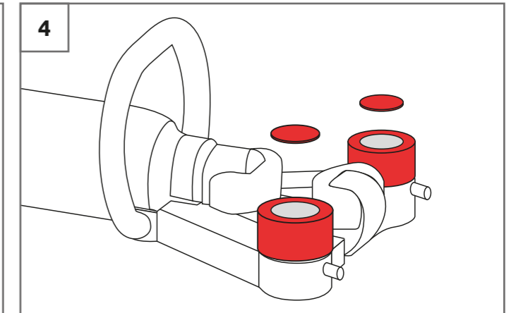
Place the protection cap on the rollers Posizionare il tappo di protezione sopra le boccole
